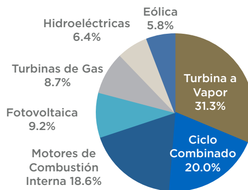
Generación bruta de electricidad por tipo de tecnología Participación porcentual (%) enero-junio 2025
